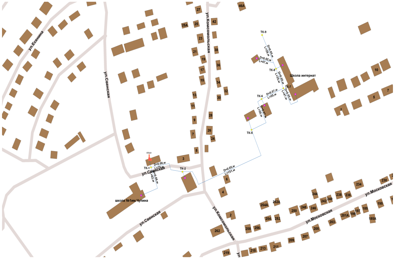
Рис.9 Схема горячего водоснабжения с. Супонево.
