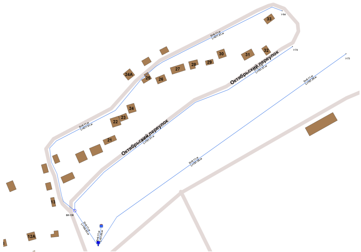
Рис.6 Схема водоснабжения д. Курнявцево.
